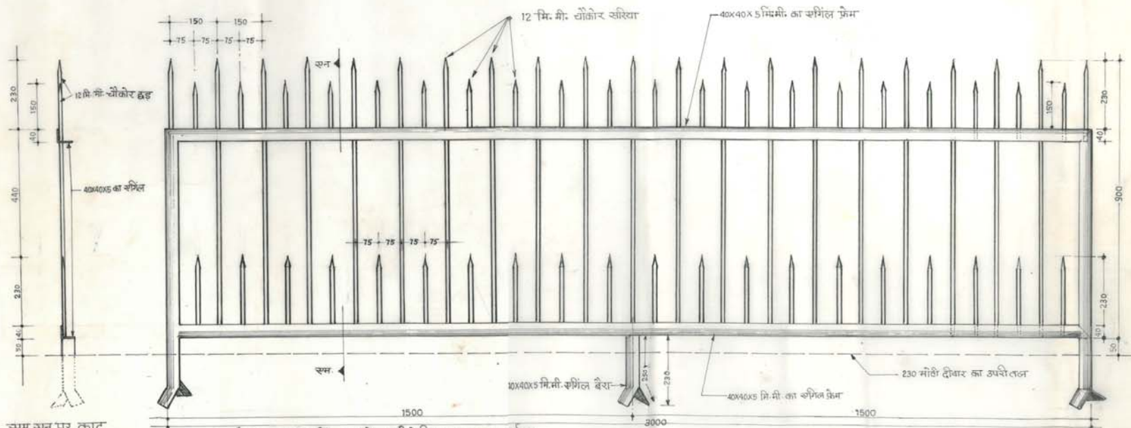
पार्क तथा बागान में लगने वाली रेलिंग का सम्मुख दृशन मापनी - 1:8
