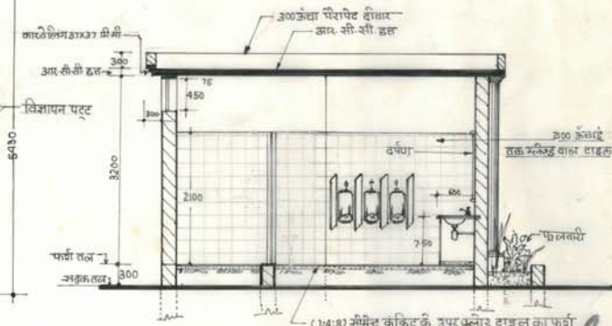
पी-पी पर काट मापनी - 1 से.मी. = 50 से.मी.
