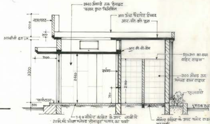
रुम-रुम पर काट मापनी - 1 से.मी. = 50 से.मी.
