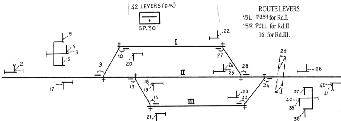
चित्र-3 (लॉकिंग सारणी 1 देखें)
