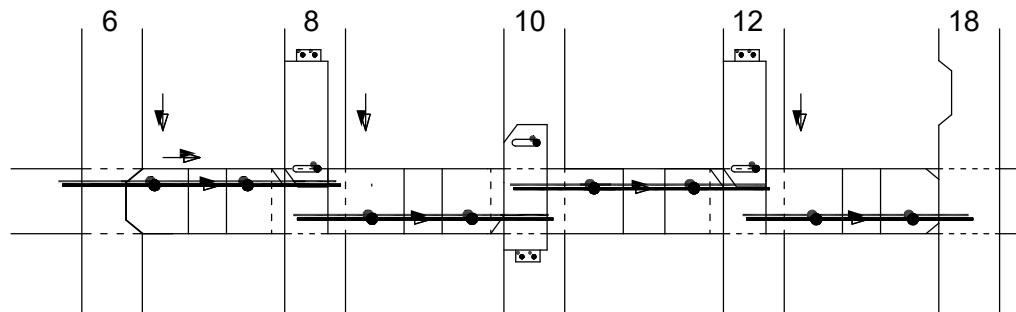
6 रिलीज्ड बाई (18W8R10N12R)
