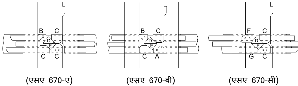
चित्र 7.4 (क) डायमंड विशेष के विभिन्न संयोजन
